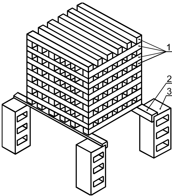
Рисунок В.1 — Устройство деревянного штабеля (модельного очага пожара класса А) для проведения огневых испытаний
