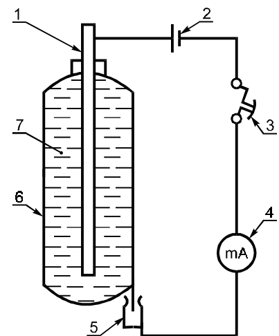
1 — электрод; 2 — стабилизированный источник постоянного тока с напряжением 3,7 В; 3 — выключатель; 4 — миллиамперметр с пределом измерения до 200 мА; 5 — жим; 6 — корпус огнетушителя; 7 — раствор электролита
